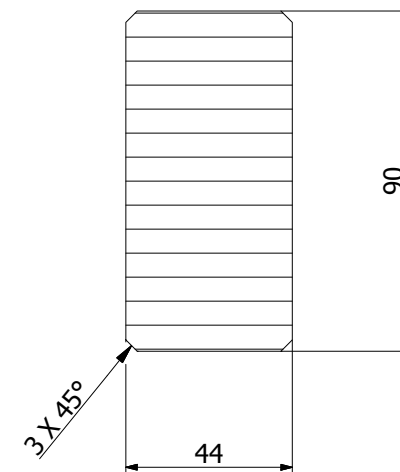
A-A ( 1 : 2 )
