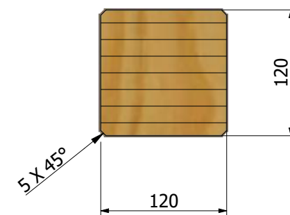
A-A ( 1 : 5 )
