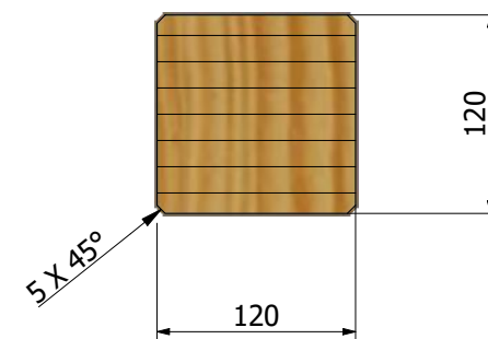
A-A ( 1 : 5 )
