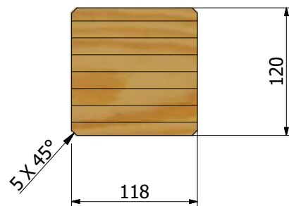
A-A ( 1 : 5 )
