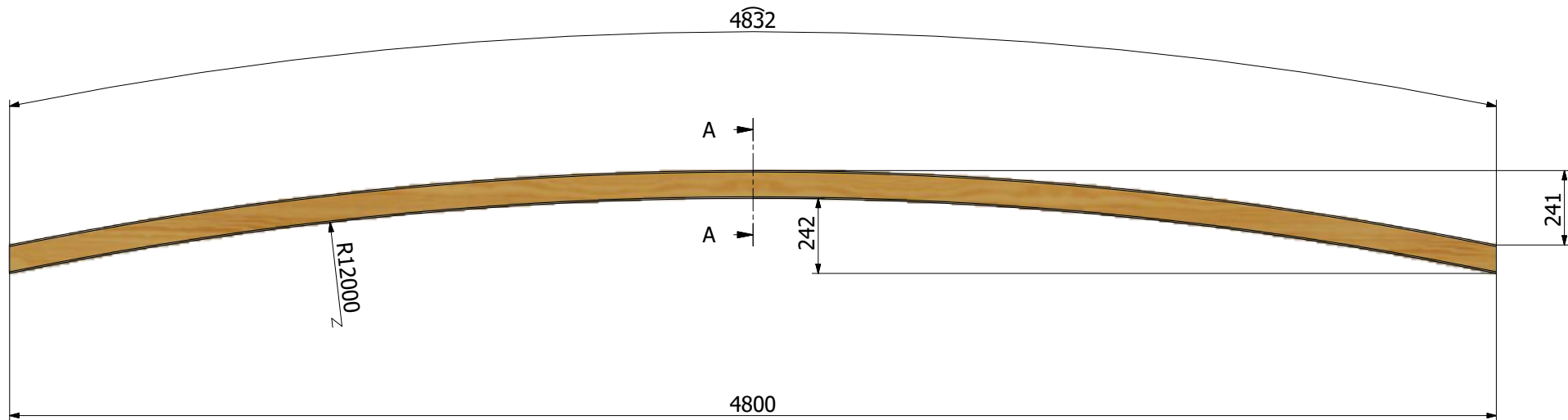
A-A ( 1 : 5 )
