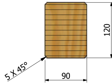
A-A ( 1 : 5 )
