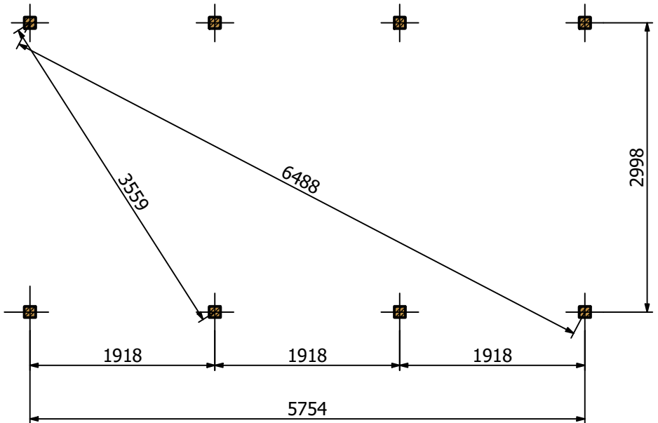
A-A ( 1 : 55 )
